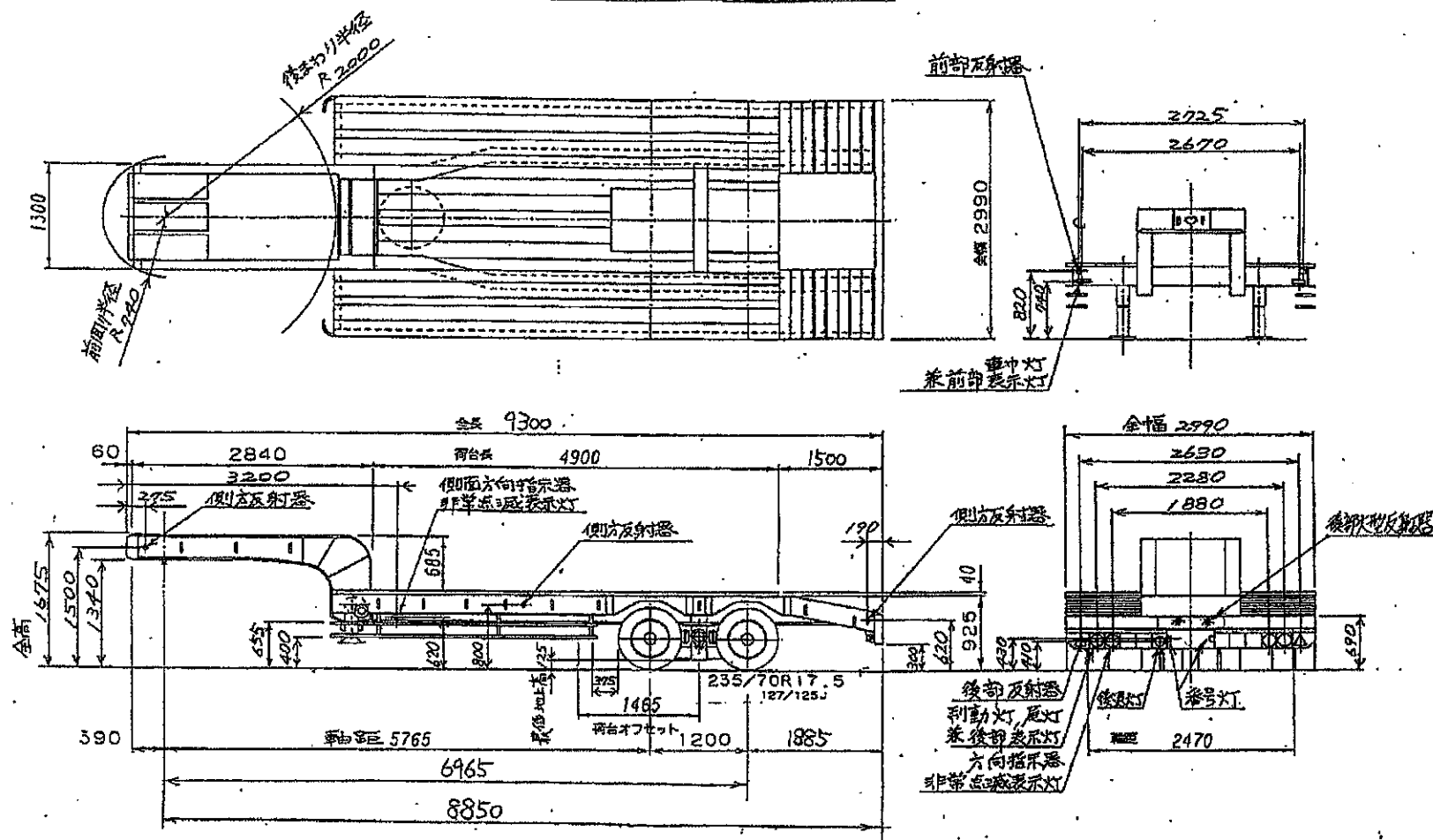
トールモービル PLR 43/AH 型 外観四面図
